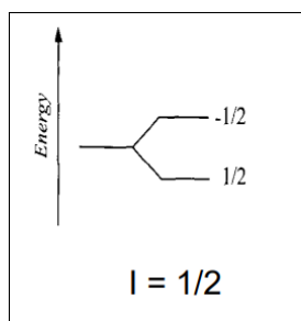
Figura 21: Stati possibili per un nucleo di spin \frac{1}{2} : \frac{1}{2} = \alpha , -\frac{1}{2} = \beta
