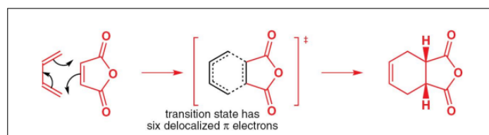
Figura 15: Reazione di Diels-Alder con TS mostrato
