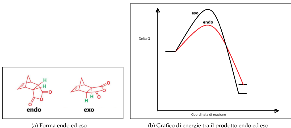
Figura 18: Confronto tra le forme endo/eso e il grafico di energie
